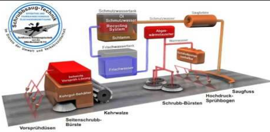
BIOTEC No1 Schematische Darstellung der Schrubbsaugtechnik der Biotec No 1 Ölspurnassreinigungs-Maschine
